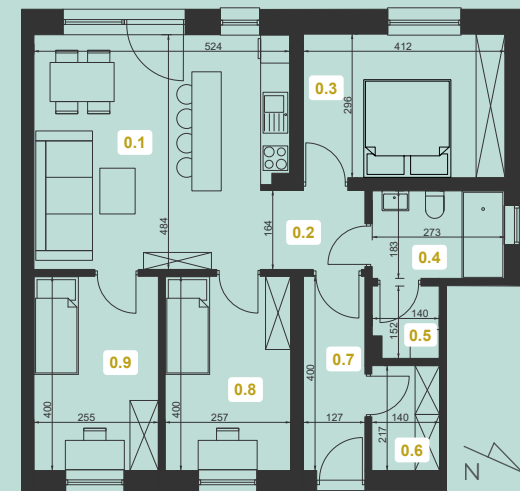
Rzut parteru
