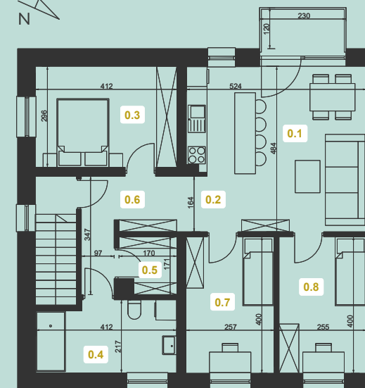
Rzut piętra
